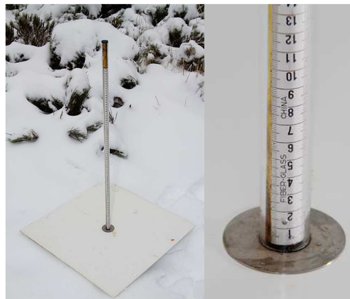
Fig. 32 Jalón y placa de nieve reciente
