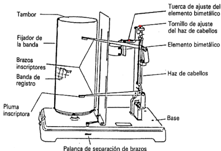
Fig. 27 Elementos del termohigrógrafo
