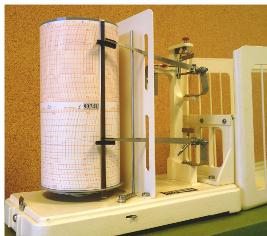
Fig. 26 Termohigrógrafo
